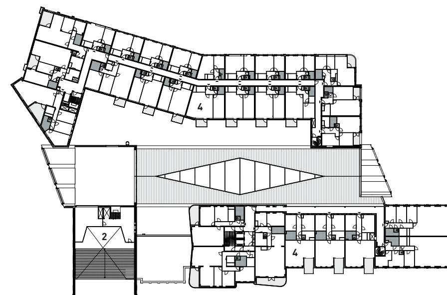
Tweede verdieping | First floor
