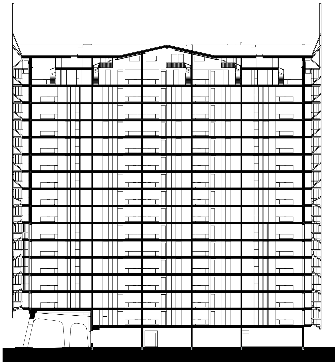
Doorsnede | Section
