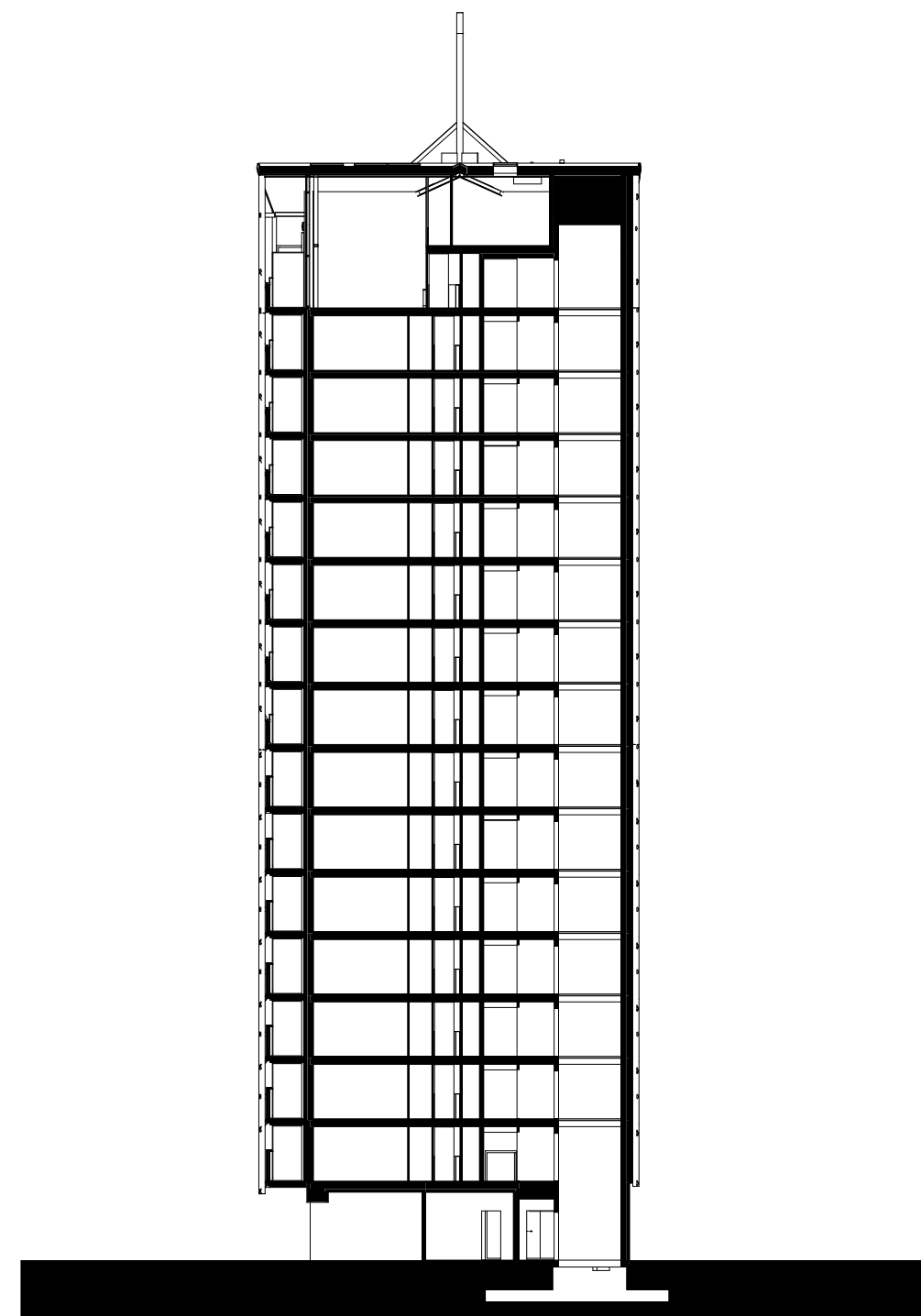
Doorsnede | Section
